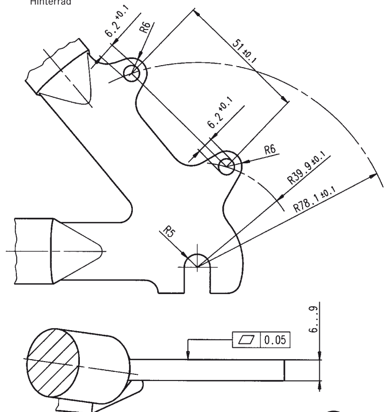
Hinterrad
