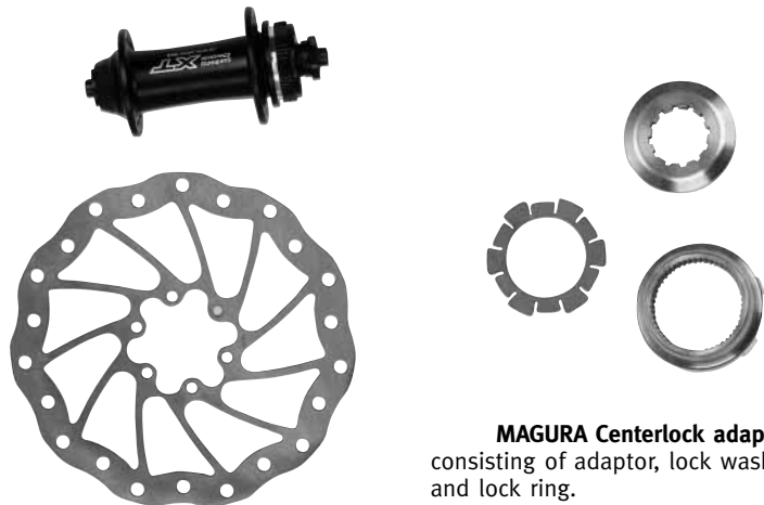
Adaptateur MAGURA Centerlock , consiste en 1 adaptateur, 1 rondelle de blocage et 1 vis de blocage.
